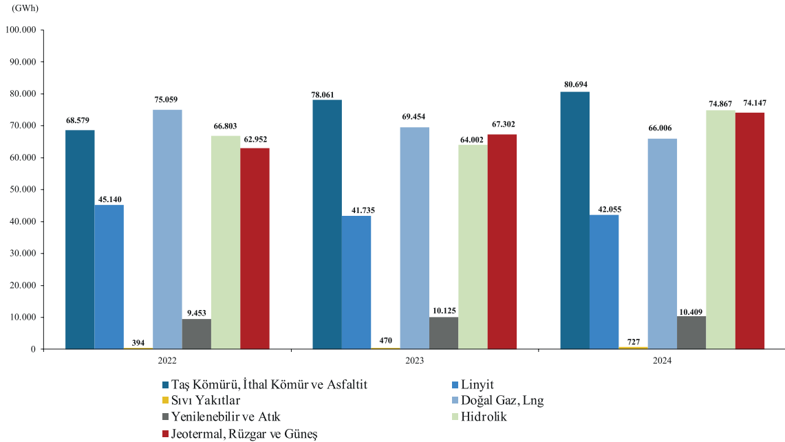
Grafik 28. Elektrik Enerjisi Üretiminin Birincil Enerji Kaynaklarına Göre Dağılımı
